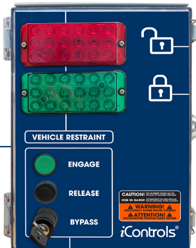
Panneau de système de retenue de véhicule avec affichage à lumières DEL Rouge et Vert
